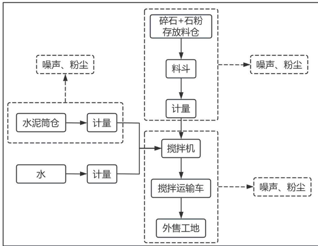
图 5-3 拌合站工艺流程图
